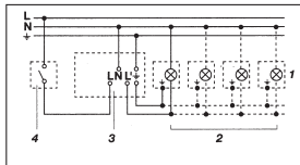
2. Belysning med befintligt nolledare
