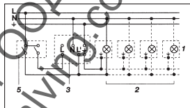
3. Priklopec preko serijskega stikala za ročno in avtomatsko delovanje
