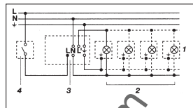
1. Valgusti ilma nulljuhtmega
