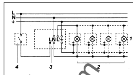
1. Nollajohtimen kytös tunnistimen kautta
