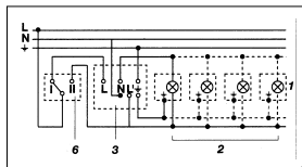
4. Připojení prostřednictvím stírávého přepínače pro trvalé osvětlení a automatický provoz
