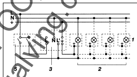
3. Prijungimas per nuoseklią jungiklį, norint įjungti rankinio ir automatinio valdymo režimą
