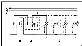
4. Sürekli ışık ve otomatik işletim için, komütatör üzerinden bağlantı Konum I: Otomatik işletim Konum II: Sürekli aydınlatma için elle işletim
