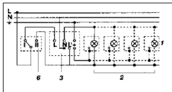
4. свързване към двоен/девиаторен прекъсвач за режим постоянно включена светлина и автоматично опериране
