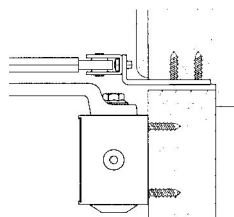
Скоба и рамо за стандартен монтаж с профилен орнамент Арт.Ном.8382/1
