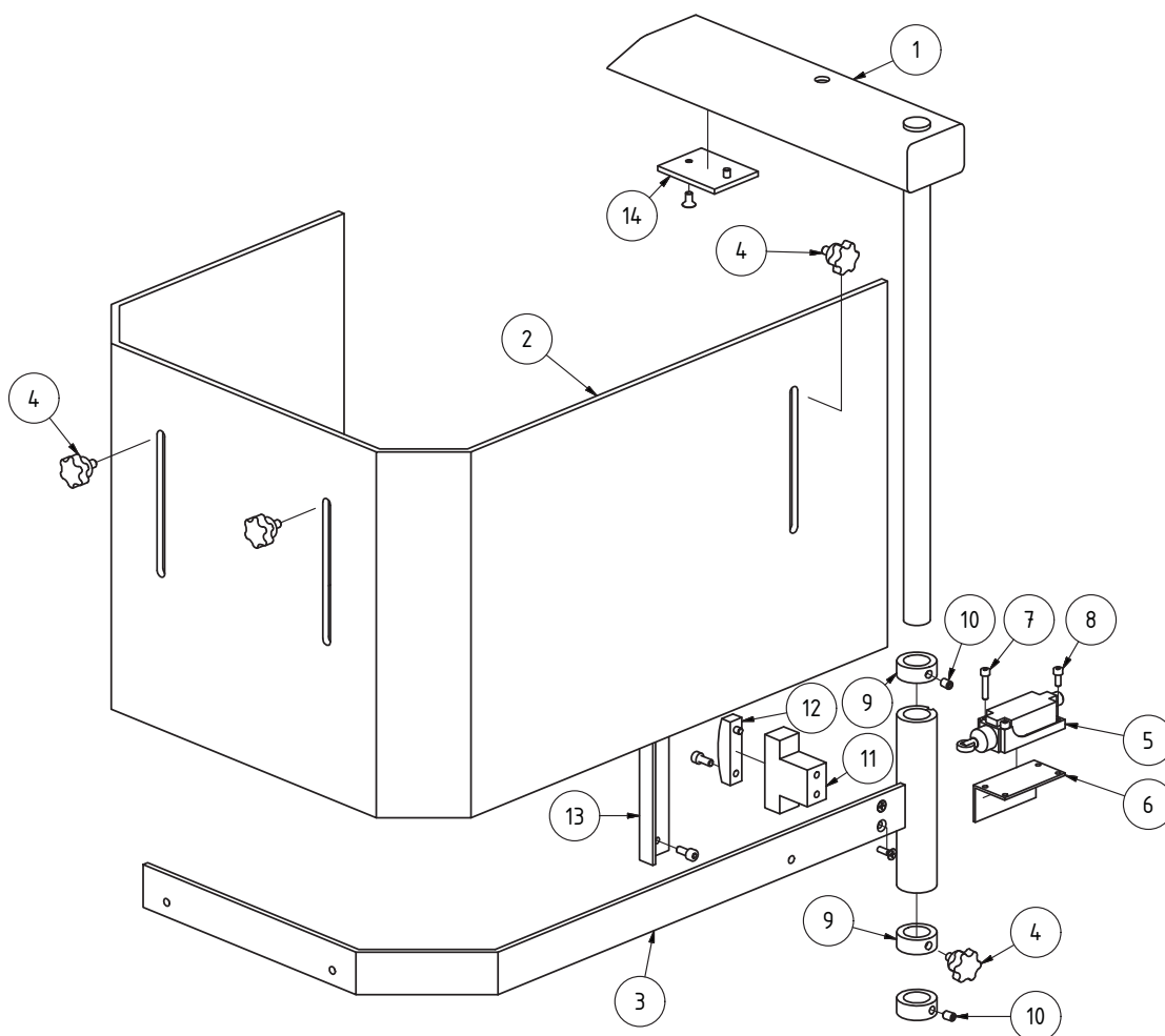
Abb. 1-24: Fräsfutterschutz - Milling chuck protection
