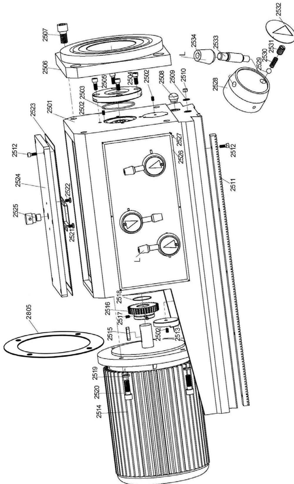
Abb.1-17: Schaltgetriebe 1 - 4
