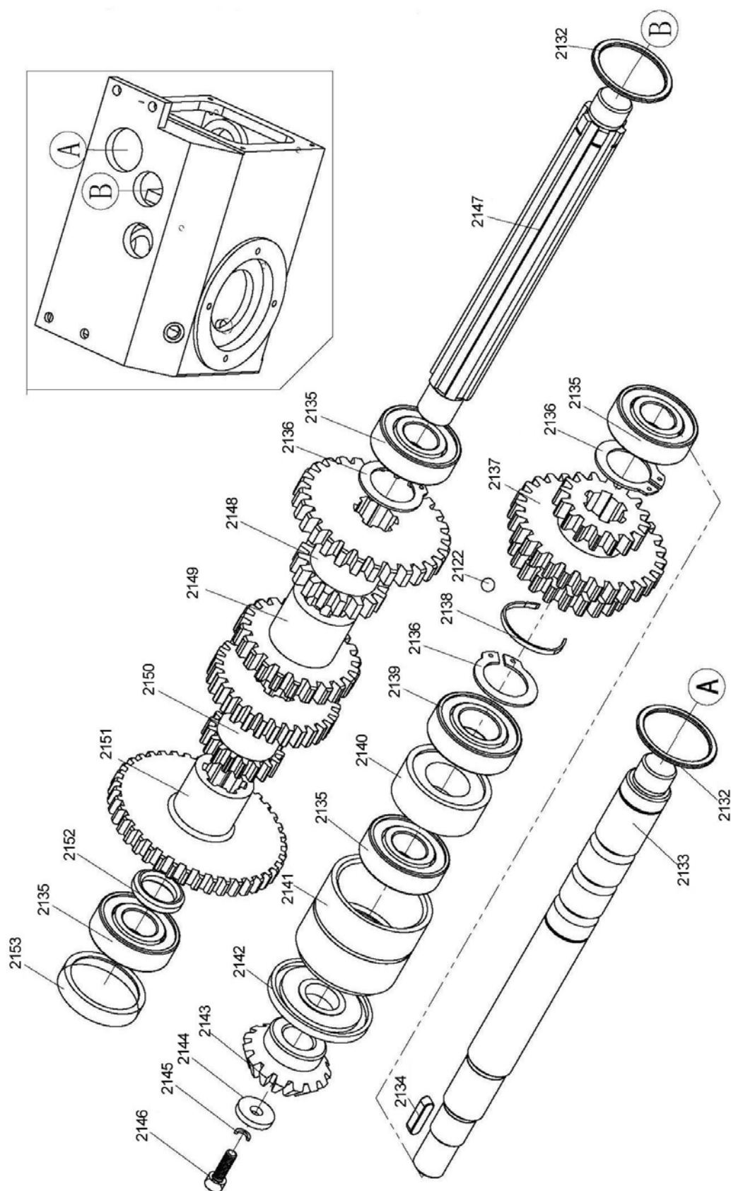
Abb. 1-14: Vorschubgetriebe 2 - 4
