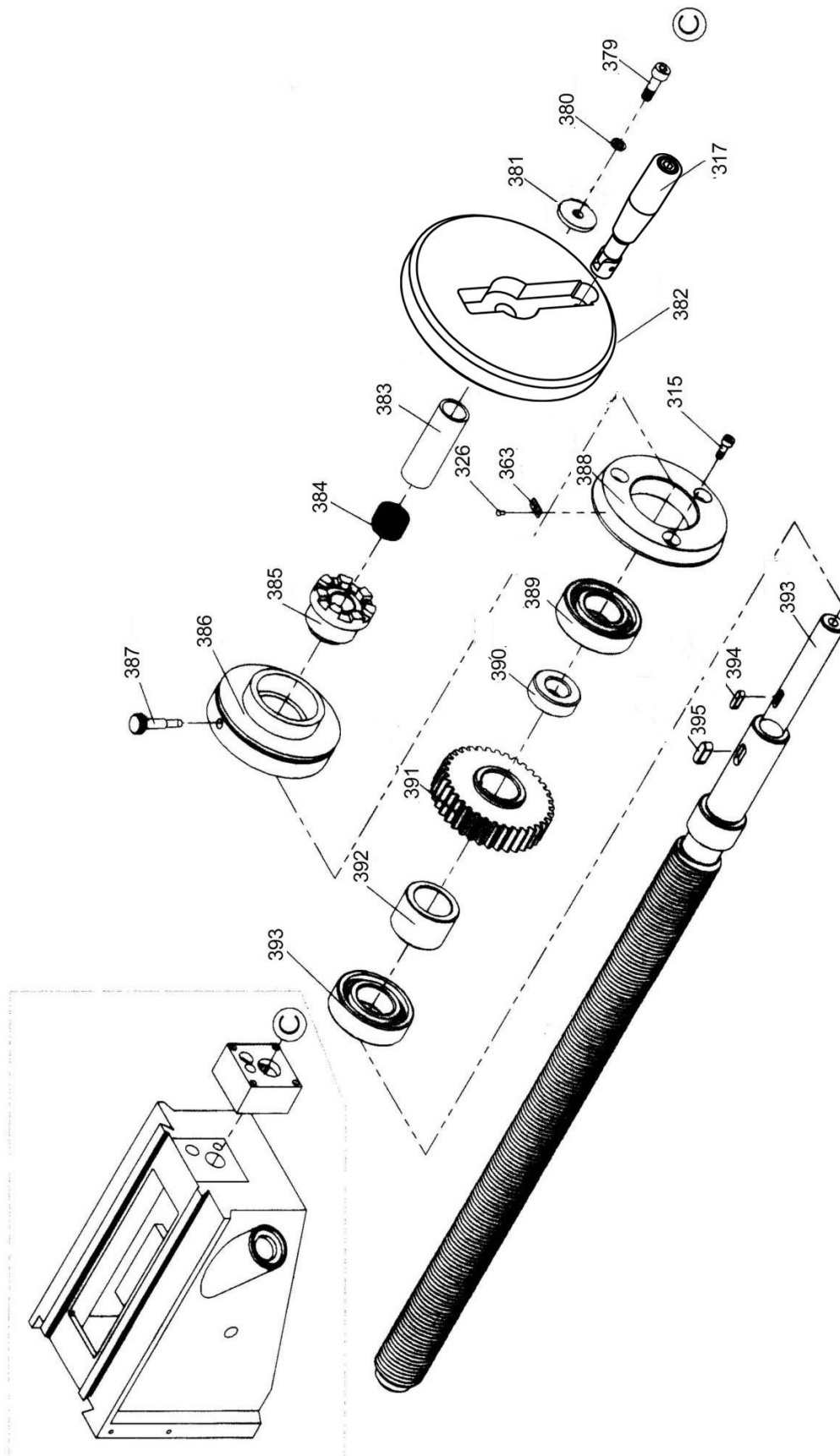
Abb. 1-4: Konsole 3 - 4
