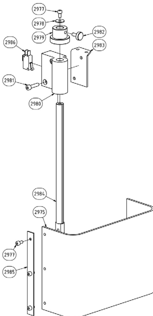
Abb. 1-22: Fräsfutterschutz - Milling chuck protection
