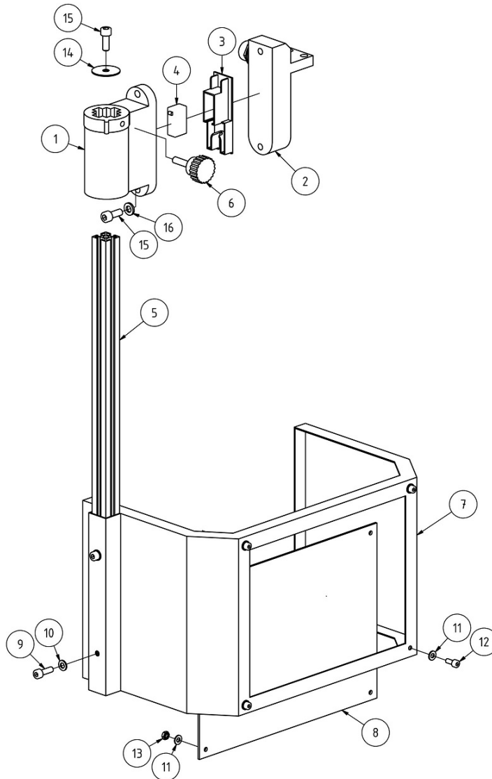
Abb. 1-23: Fräsfutterschutz - Milling chuck protection
