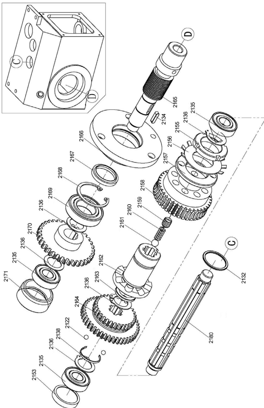
Abb. 1-16: Vorschubgetriebe 4 - 4
