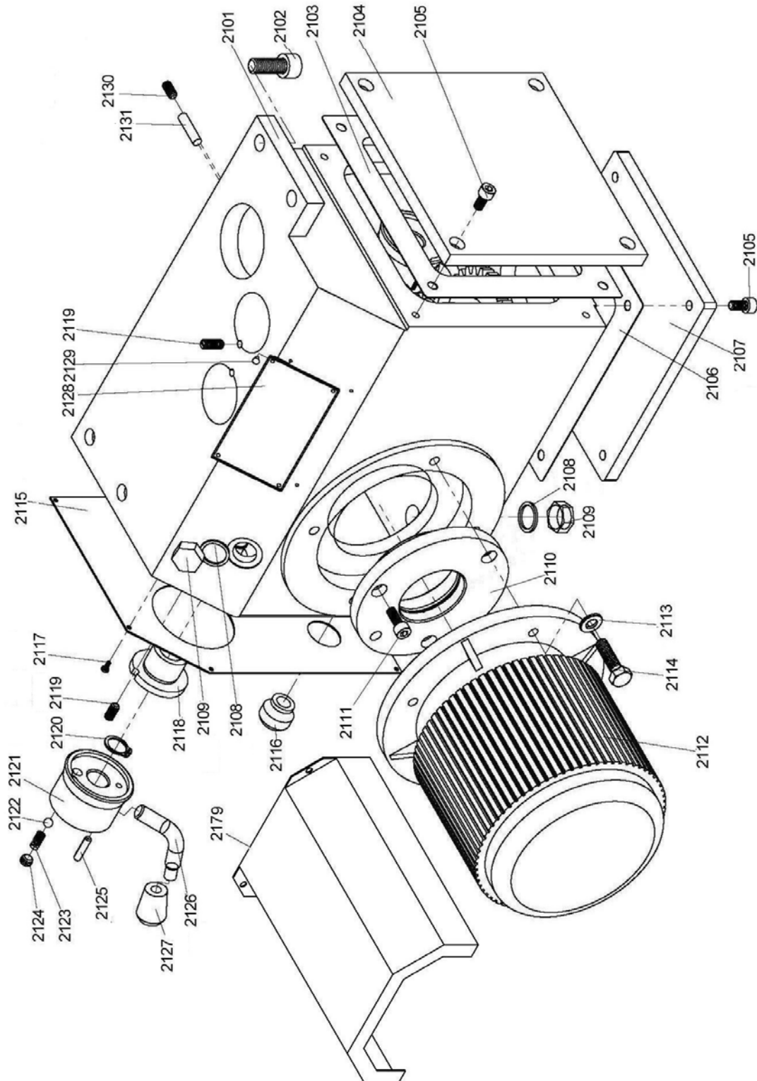
Abb. 1-13: Vorschubgetriebe 1 - 4
