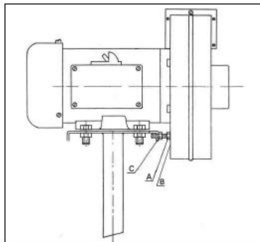
Фигура 12 – Регулиращ болт
