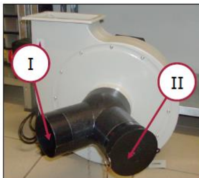
Фигура 13 – Свързване на смукателната тръба
