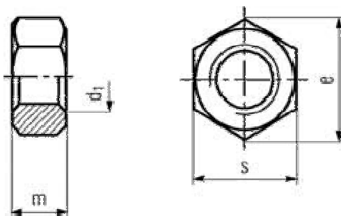
DIN 934 - Гайка шестостенна
