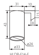
HLDR-E14-F
