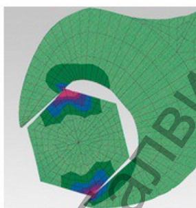
Традиционен гаечен ключ: Притискането на ръбовете води до повреди
