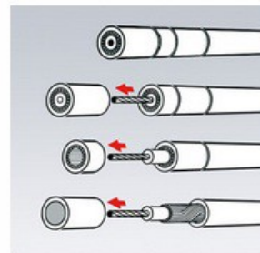
Тристепенно сваляне на изолацията на коаксиален кабел
