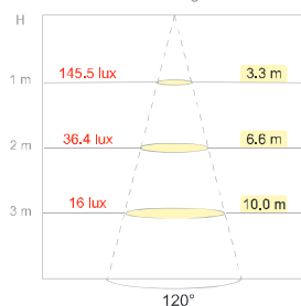
Светлинен конус (20W) Cone Diagram
