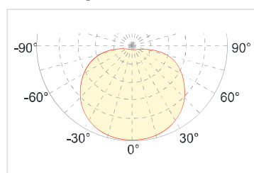
Светлоразпределителна крива Light Distribution Curve
