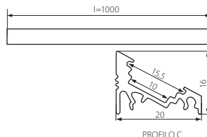
PROFILO C
