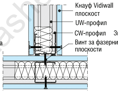
W361-C1 Т-връзка
