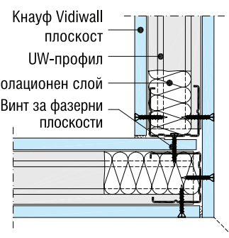
W361-D1 Ъгъл
