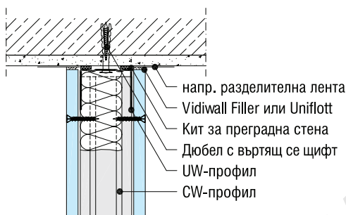
W361-V01-A Връзка към таван
